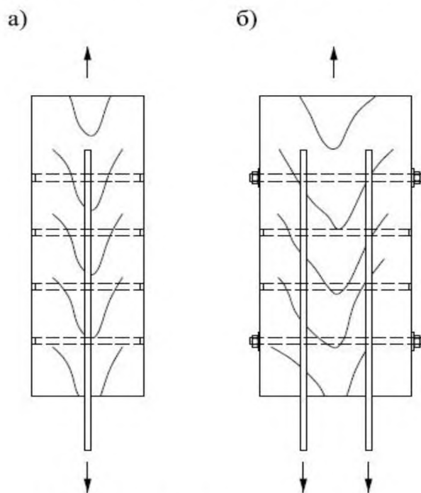
Рисунок 2 — Нагельные соединения с накладками
