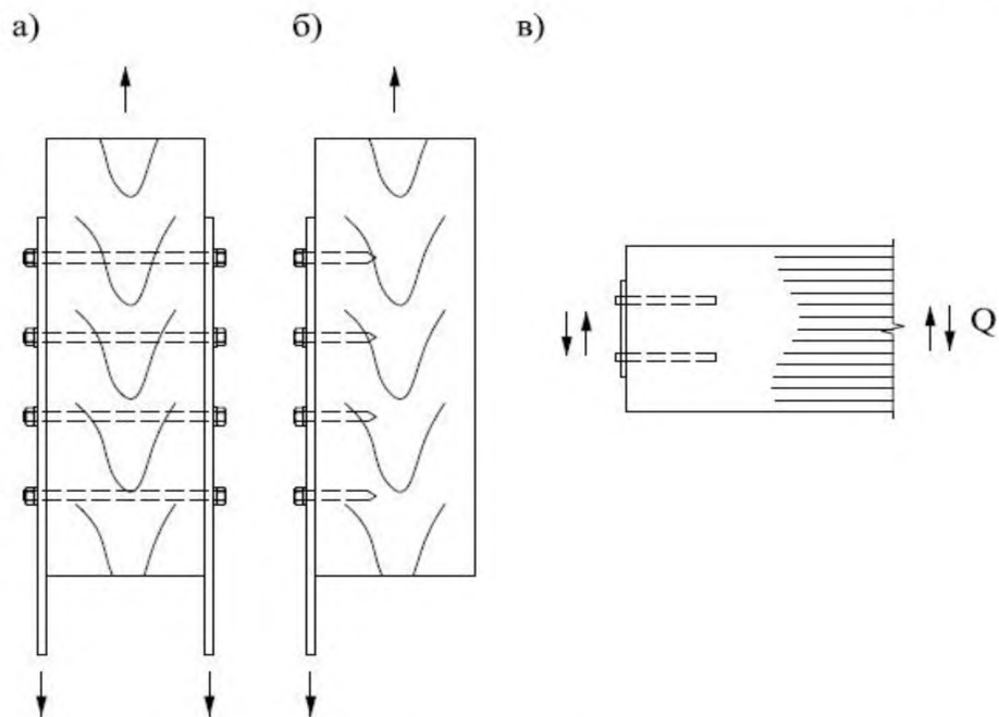
Рисунок 2 — Нагельные соединения с накладками
